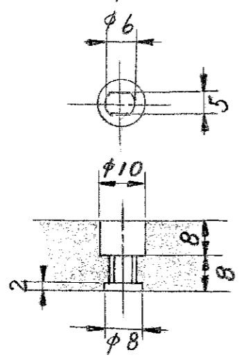
取付穴部詳細
