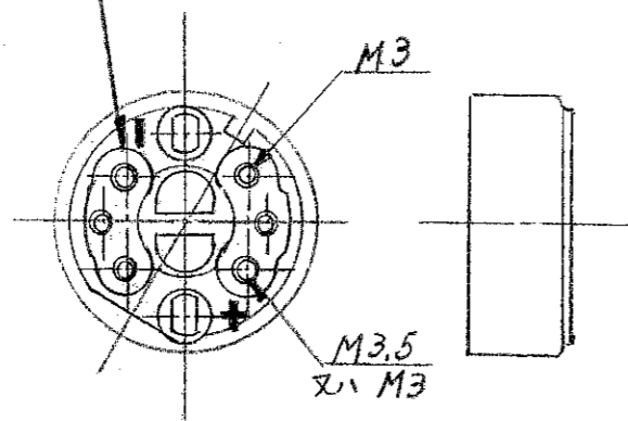
外部蓋裏面図
