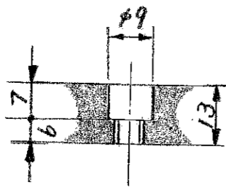
取付ヶ穴部断面
