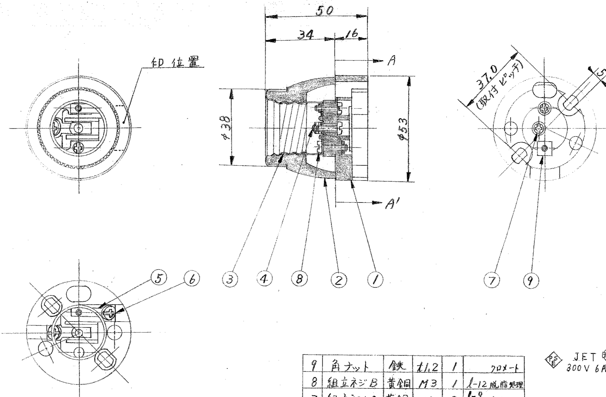
A-A' (カバーを取り上ヨリ見ル)
