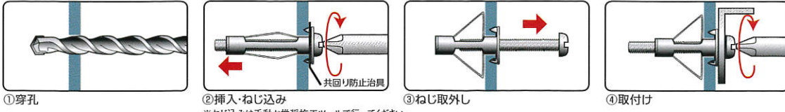
①穿孔 ②挿入・ねじ込み ※ねじ込みは手動が推奨施工ツールで行ってください。 ③ねじ取外し ④取付け
