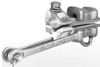
アルミ線用引留クランプ
