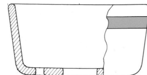
塩風受皿 ピン碍子と一緒に ご使用ください。
