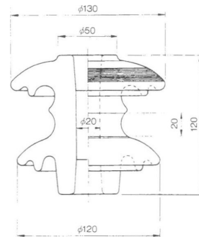
高圧引留碍子
