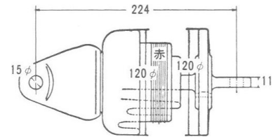
高圧耐塩耐張碍子
