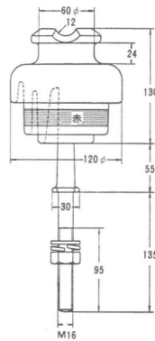
高圧耐塩ピン アーム/アングル
