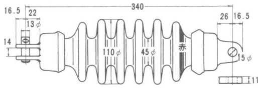
高圧中実耐張碍子
