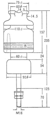
高圧中実碍子
