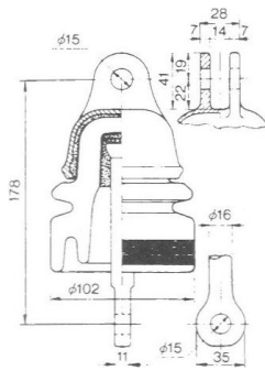
高圧耐張碍子 直角/平行
