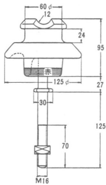
高圧ピン碍子 アーム/アングル
