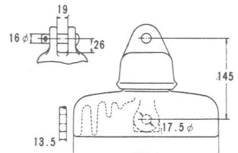
250EP-F(耐塩型)
