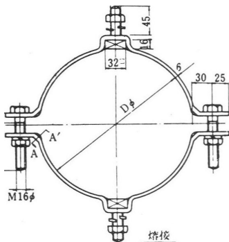
電柱バンド A型
