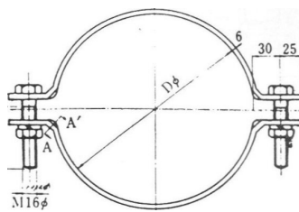
電柱バンド B1型
