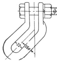
変形クレビス
