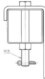
JR碍子金具用真棒
