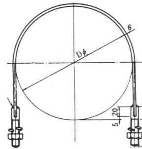
電柱バンド C型
