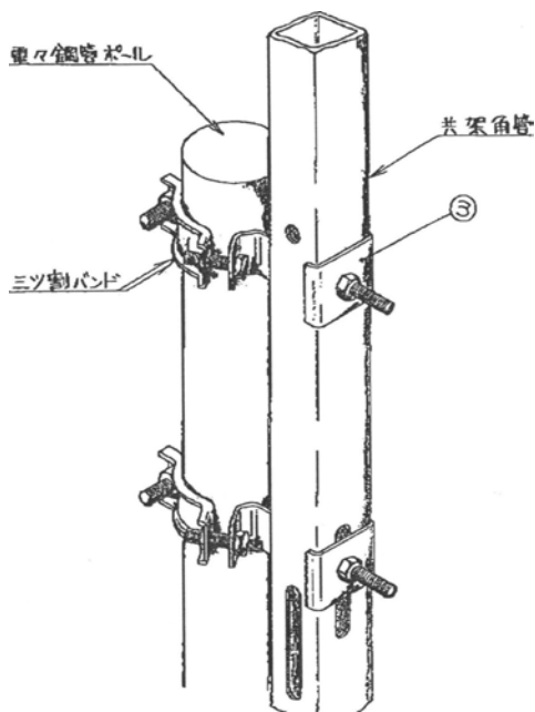
三ツ割バンド組付状況
