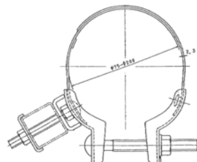
共架角管取付バンド 75~200φ
